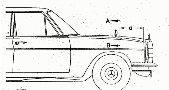
Bild 59-1/2 Anordnung Außenspiegel rechts ab 8/69 (bei Rechtslenker-Fahrzeugen spiegelbildlich links)
