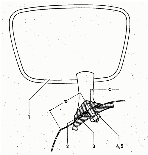
Bild 59-1/3 Schnitt A-B: Befestigung Außenspiegel am Vorderkotflügel 1 Außenspiegel 2 Unterlage 3 Gegenplatte 4 Federring 5 Sechskantmutter
